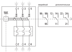
ВА-99М 400А-1250А
