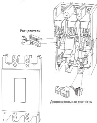
ВА-99М 63А-250А
