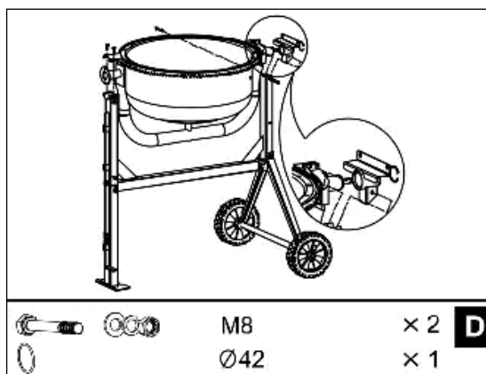
Рис. 20. Установка нижнего полубака
