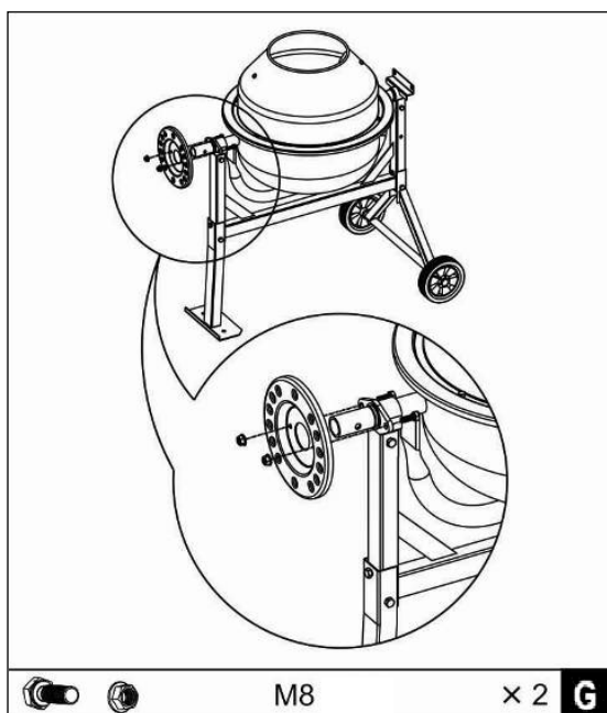
Рис. 23. Диск фиксатор
