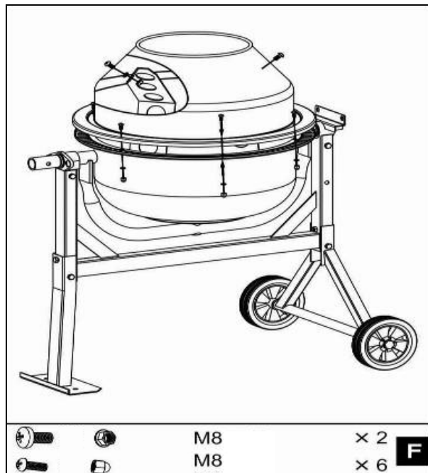
Рис. 22. Установка лезвий и верхнего полубака
