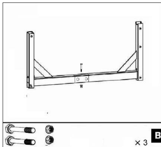
Рис. 6. Сборка рамы
