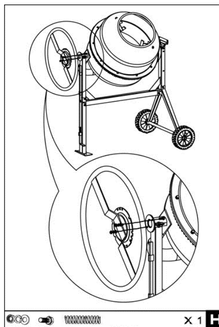
Рис. 24. Поворотное колесо
